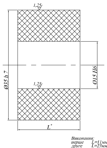
Рис. 7 – Робоче креслення втулки
