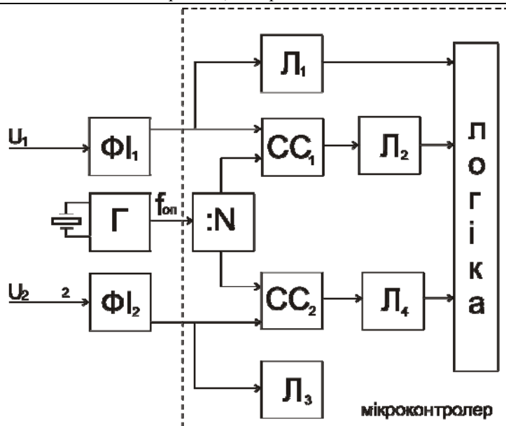
Рис. 4. Структурна схема лабораторного макету фазометра з використанням мікроконтролера (для 3-х різних методів)
