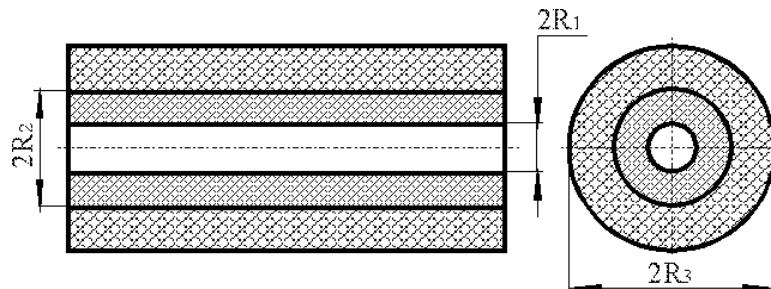
Рис. 3. ЕРЕ, оточений рівномірним шаром компаунду
