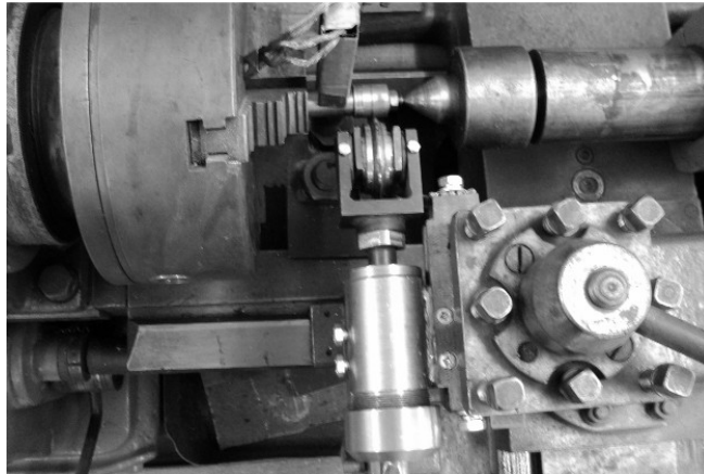
Рис. 3 – Вигляд процесу обробку ЕМО циліндричної заготовки на базі токарного верстату
