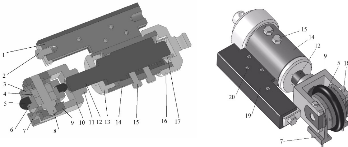
Рис. 2 – Буда пристрою для електромеханічного зміцнення
