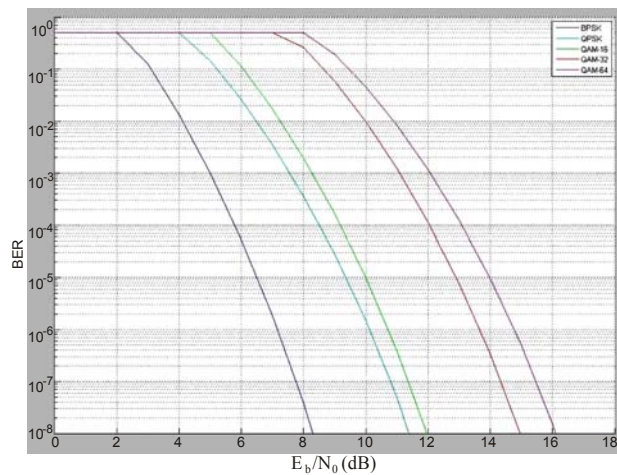
Рис. 5. Криві залежності BER від SNR для різних типів модуляцій для каналу з SISO
