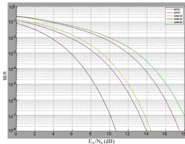
Рис. 4. Криві залежності BER від SNR для різних типів модуляцій для каналу з SISO
