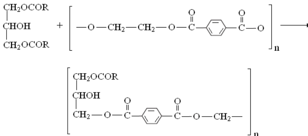
Рис. 1. Взаємодія ацилгліцеролу природного жиру та поліетилентерфталату
