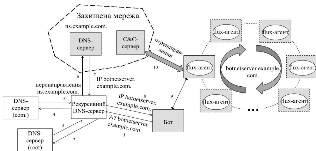
Рис. 7. Схема функціонування однопоточної «швидкозмінної» мережі
