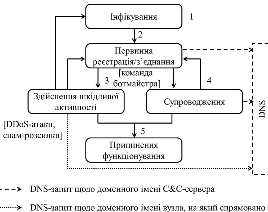
Рис. 1. Схема життєвого циклу бот-мережі з врахуванням системи доменних імен
