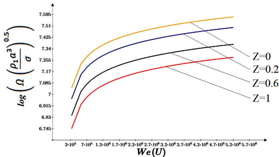
Рис. 4. Довжина хвилі у найбільш нестабільній поверхневій хвилі проти числа Вебера, We_2 , як функція числа Z
