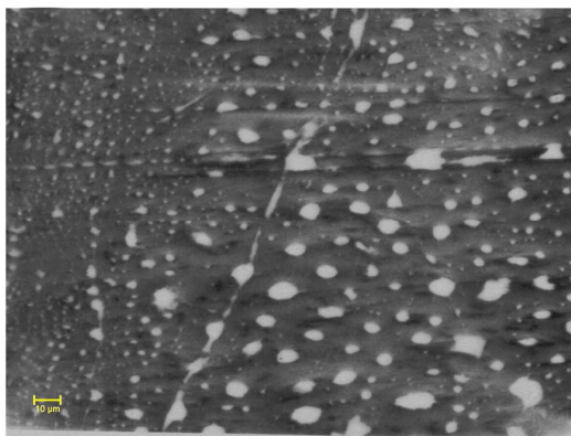
Рис.1. Зображення структури окисної плівки на поверхні кристалів кремнію, отримане методом растрової електронної мікроскопії зразу після завершення магнітної обробки.
