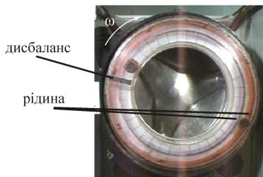
Рисунок 2.3 - Розміщення рідини при частоті обертання ротора \omega=70 \text{ c}^{-1}
