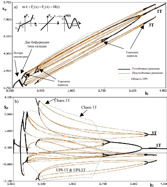
Рис. 1. Бифуркационная диаграмма для трилинейной симметричной системы с линейным вязким трением при изменении амплитуды внешнего гармонического воздействия. На диаграммах отображены бифуркационные группы 1Т и 3Т. Показаны значения перемещения (а) и скорости (б) неподвижных точек устойчивых и неустойчивых периодических решений.
