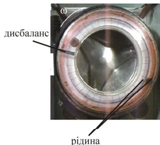
Рисунок 2.4 - Розміщення рідини при частоті обертання ротора \omega=93 \text{ c}^{-1}
