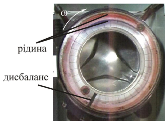
Рисунок 2.1 - Розміщення рідини при частоті обертання ротора \omega=24 с -1
