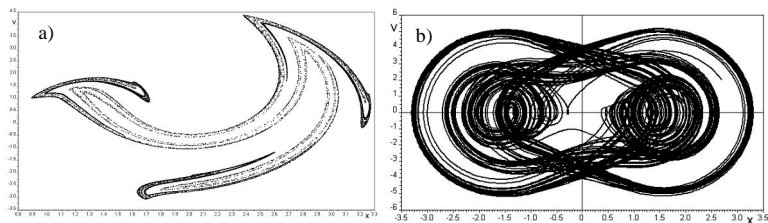
Рис. 2. Хаотический аттрактор в области с бесконечным числом неустойчивых режимов UPI бифуркационных групп 1Т и 3Т на плоскости Пуанкаре за 50000 периодов внешнего воздействия (а) и его фазовый портрет (100 периодов, б). Трилинейная симметричная система с турбулентным трением (кубическая характеристика) при внешнем гармоническом воздействии.
