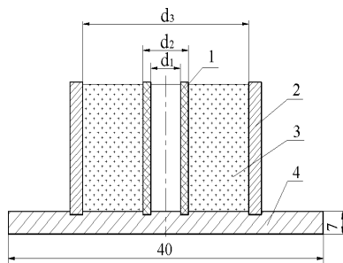
1 - керамическая трубка резистора; 2 - полый стальной цилиндр; 3 - компаунд; 4 - опорная пластина. Рис. 3. Схема приспособления для определения физико-механических характеристик керамики резисторов
