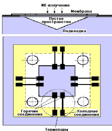
Рис. 3. Схема конструкции теплового сенсора на термопарах.
