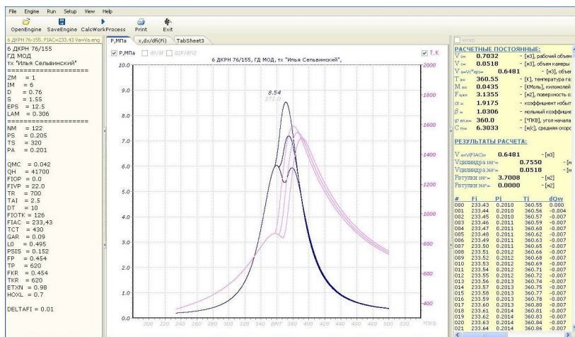
Рисунок. Интерфейс программы расчета рабочего процесса с учетом динамики тепловыделения по методу В.С.Семенова и В.И.Квятковского
