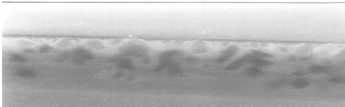
Рис. 1. Профиль пористых дефектов в протравленном слое кремния. Масштаб 1:100000.
