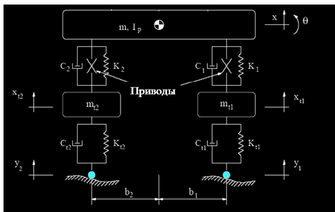
Рис. 1 Структурная схема управляемой подвески
