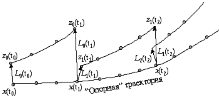
Рисунок 1 — К определению экспоненты Ляпунова из значений временного ряда
