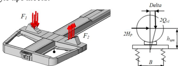
Рис. 1. Модель рамы вагона-цистерны и схема приложенных нагрузок от боковой силы 2H_p .
