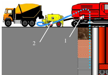
Рис.1. Схема заливки фибробетона
