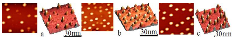
Рис. 1. АСМ-изображение (вид сверху и в пространстве) саморганизованных наностроек, которые были выращены при температуре 705^{\circ}\text{C} , 22,4 кГц, 18,6 кВт/м 2 . Номинальная толщина эпитаксиального слоя Ge составляла: (а) 6 МС; (b) 8 МС; (с) 12 МС.
