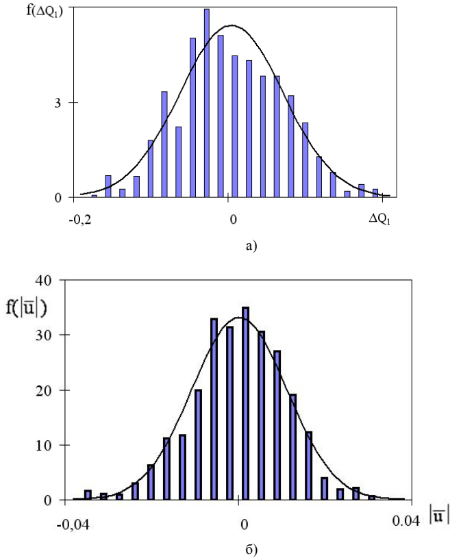
Рисунок 1 – Законы распределения случайных динамических составляющих гидротранспортного трубопровода
