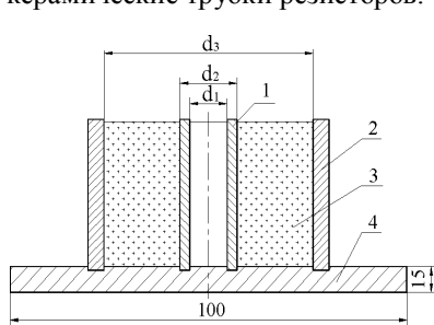
1 - полый медный цилиндр; 2 - полый стальной цилиндр; 3 - компаунд; 4 - опорная пластина. Рис. 2. Схема приспособления для определения физико-механических характеристик компаунда
