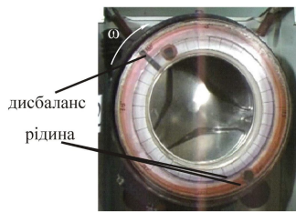
Рисунок 2.2 - Розміщення рідини при частоті обертання ротора \omega=37 с -1
