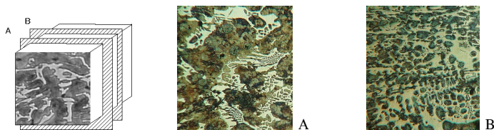
Рисунок 1 – Структура перколяционных кластеров: А и В – соответствующие сечения.
