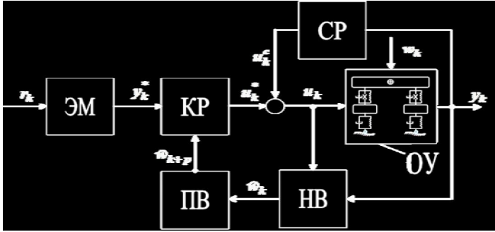
Рис. 2. Структура селективно-инвариантной системы управления гашением колебаний
