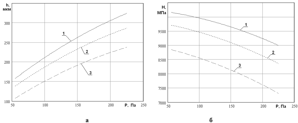
Рис. 3 – Залежність товщини азотованого шару (а), твердості поверхні (б) сталі ШХ15 від тиску в вакуумній камері в процесі дифузійного насичення при різних кількостях аргону в насичуючому середовищі: 1 – 35 % Ar; 2 – 50 % Ar; 3 – 65 % Ar
