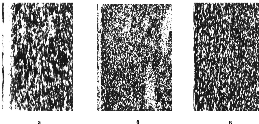
Рис. 1 – Мікроструктура сталі ШХ15 (x500) після азотованого в тліючому розряді в безводневих середовищах: а, б – з нітридною зоною різною товщиною; в – без нітридної зони
