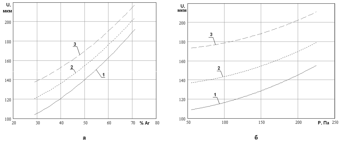
Рис. 6 – Залежність зносу сталі ШХ 15 від вмісту аргону (а) і тиску (б) в насичуючому середовищі (N 2 +Ar):
