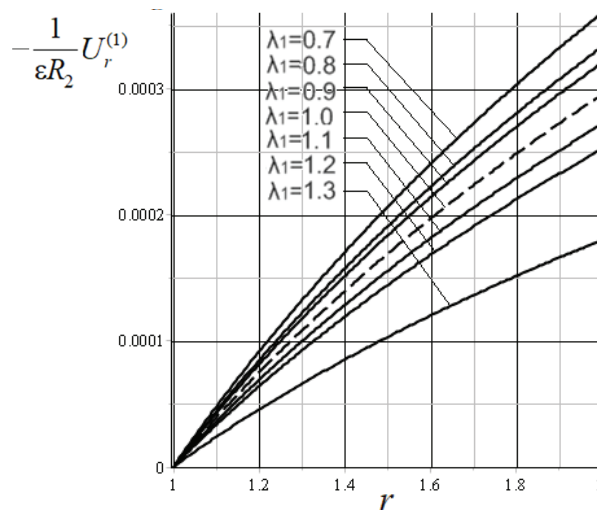
Рис. 1. Контактні переміщення -\frac{1}{\varepsilon R_2} \tilde{U}_r^{(1)} під кільцевим штампом
