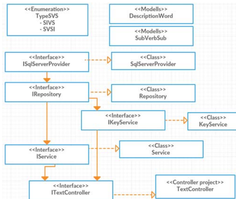
Рис. 9. Діаграма класів системи
