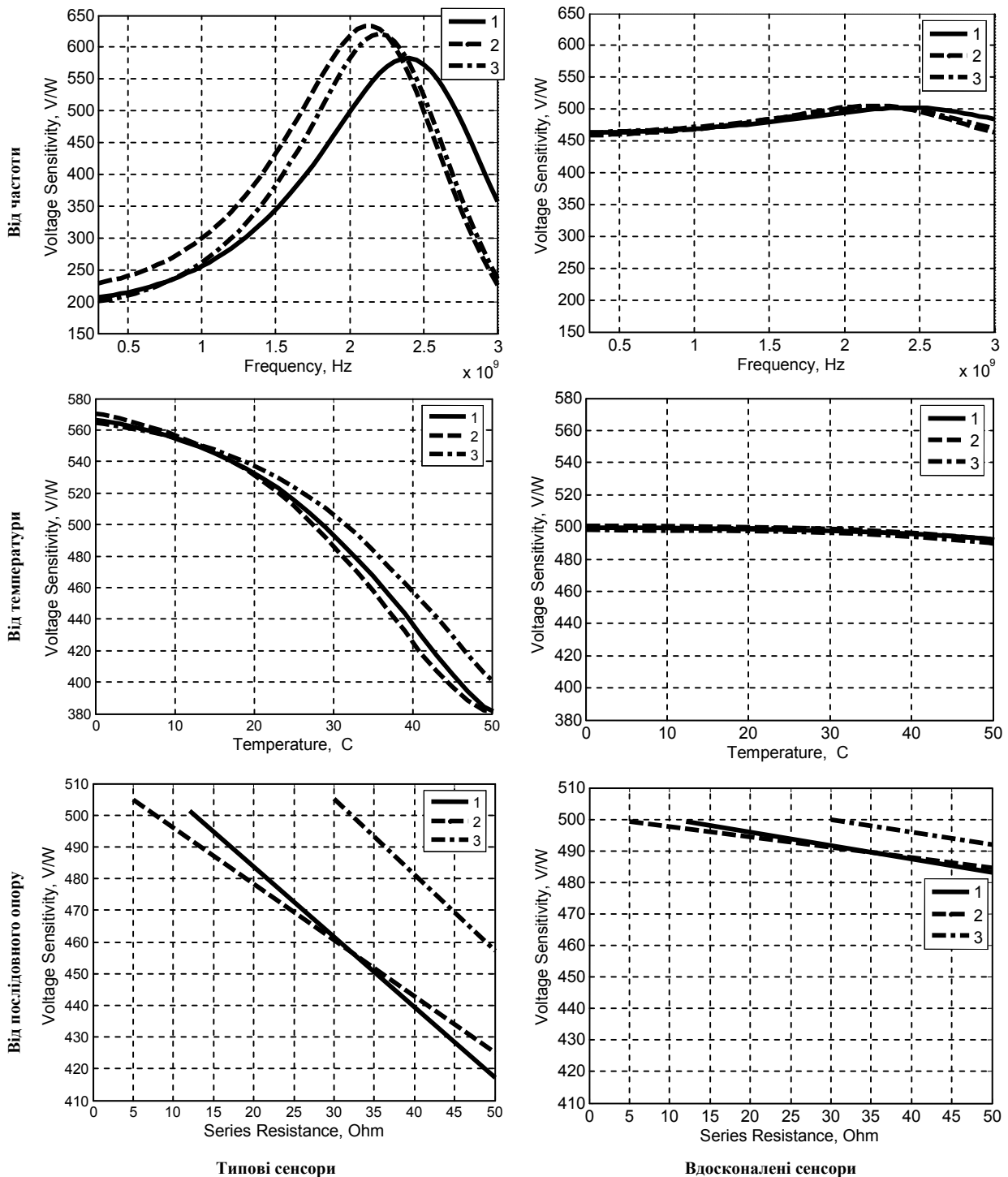
Рис. 5. Залежність чутливості за напругою від дестабілізуючих факторів
