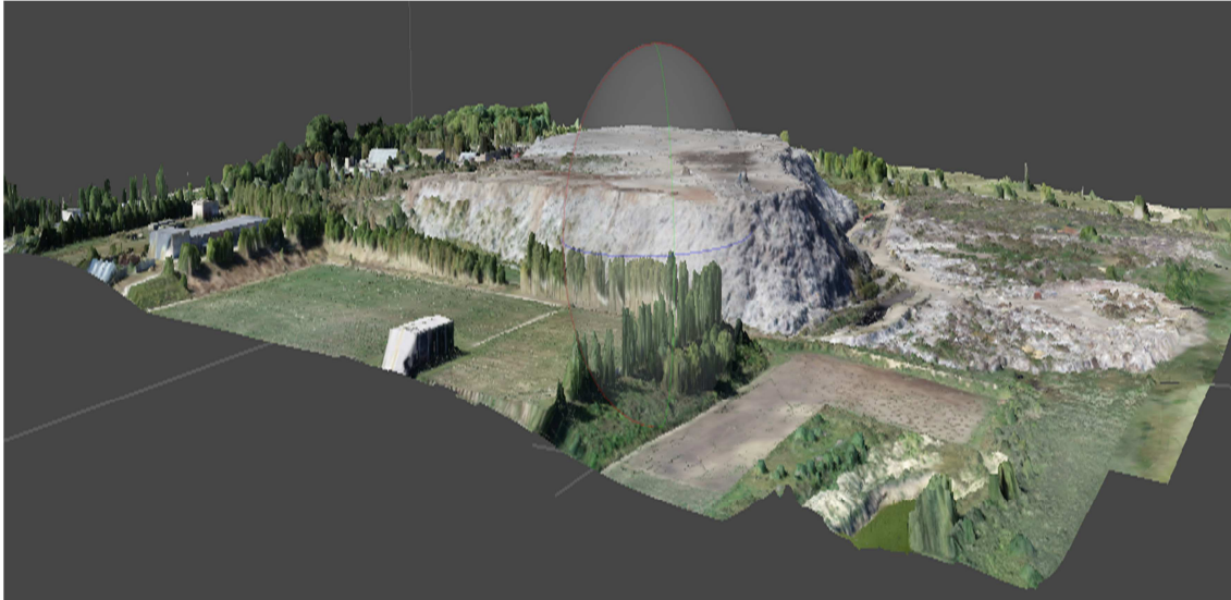
Мал. 1. Тайлова модель території знімання (Зд-модель) Хмельницького полігону твердих побутових відходів
