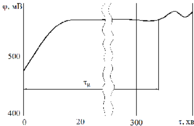
Рис. 2 – Кінетика зміни потенціалу хромованого покриття при кавітації в 3 %-му розчині хлориду натрію (сталь 45, товщина карбідної зони h_s = 91 мкм)
