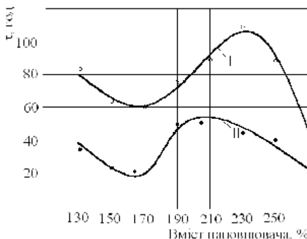
Рис. 4 – Залежність загальної довговічності \tau_{\text{заг}} (1) і часу пробою \tau_n (2) від вмісту наповнювача, %
