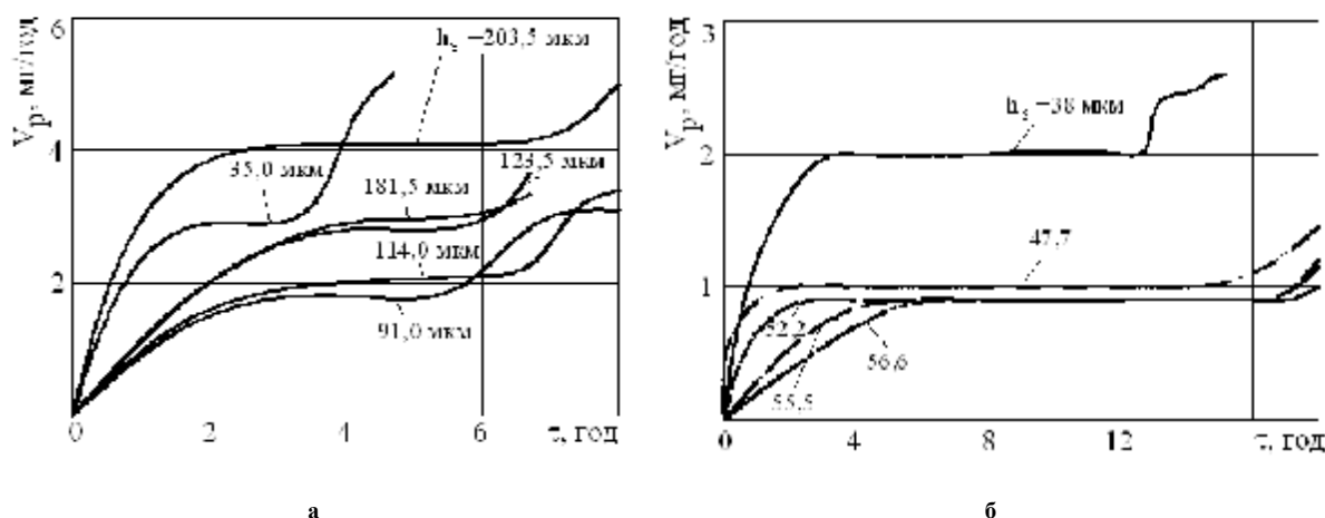
Рис. 1 – Кінетика зміни швидкості руйнування v_p теродифузійно хромованого покриття на сталі 45 (а) та сірого чавуну СЧ20 (б) в 3 %-му розчині хлориду натрію залежно від товщини карбідної зони h_k покриття
