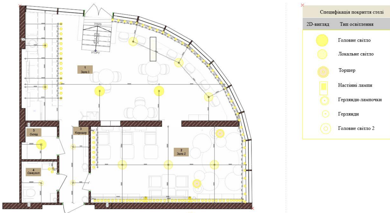
Рисунок 1.6 – План освітлення простору
