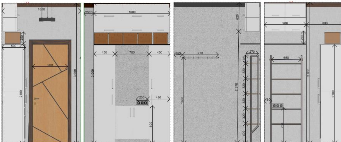
Рисунок 2.18 – Розгортка стін складу
