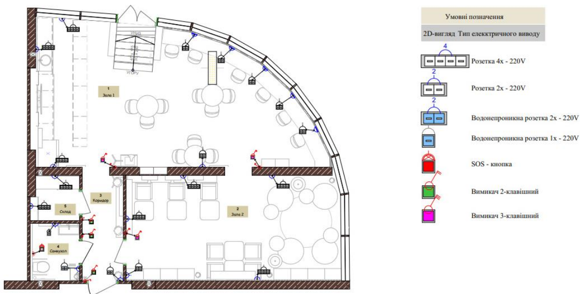
Рисунок 2.10 – План електрики
