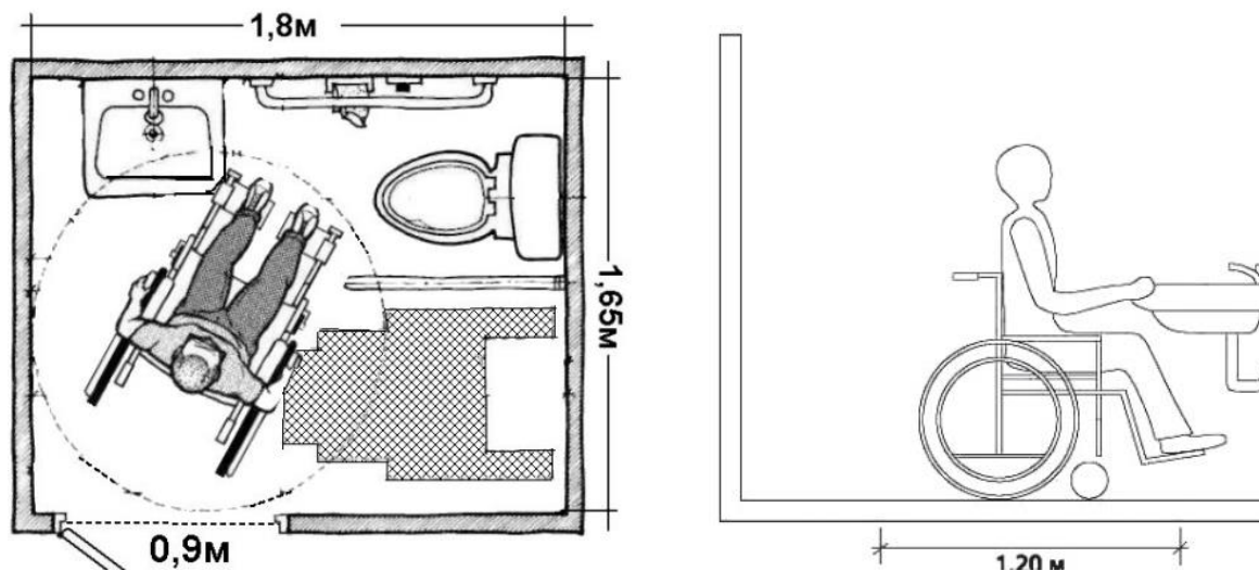
Рисунок 1.8 – Схема інклюзії в санвузлі
