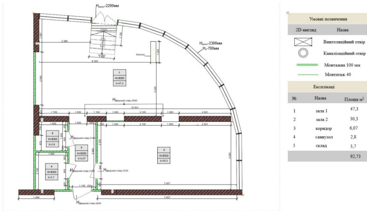
Рисунок 2.8 – План монтажу
