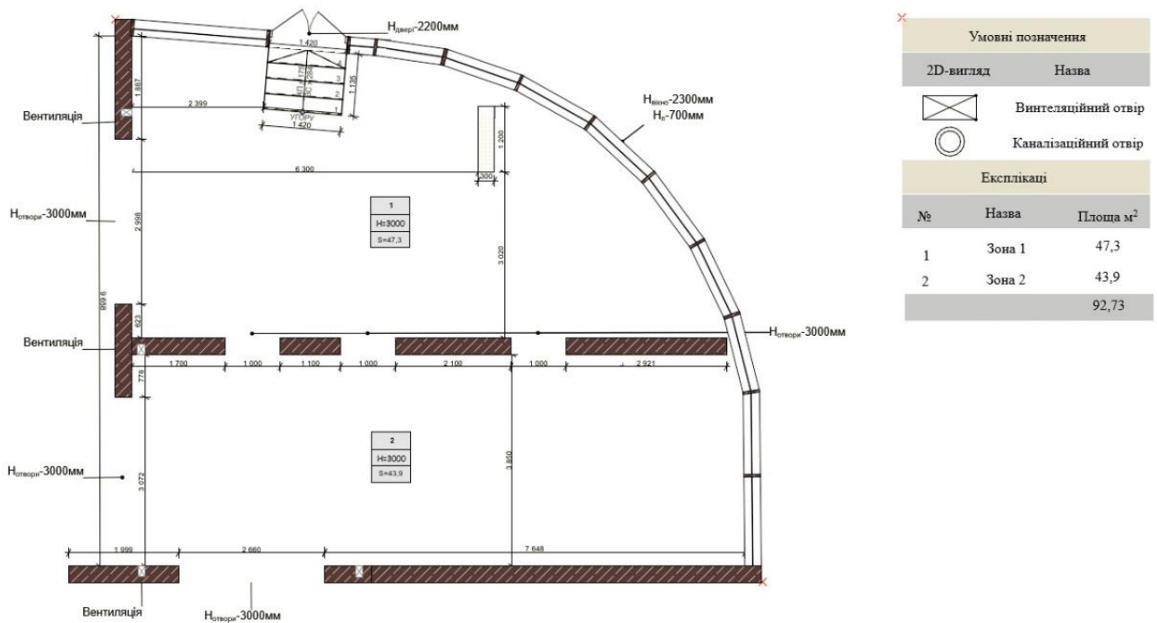
Рисунок 1.4 – Обмірний план приміщення Кафе-книгарні
