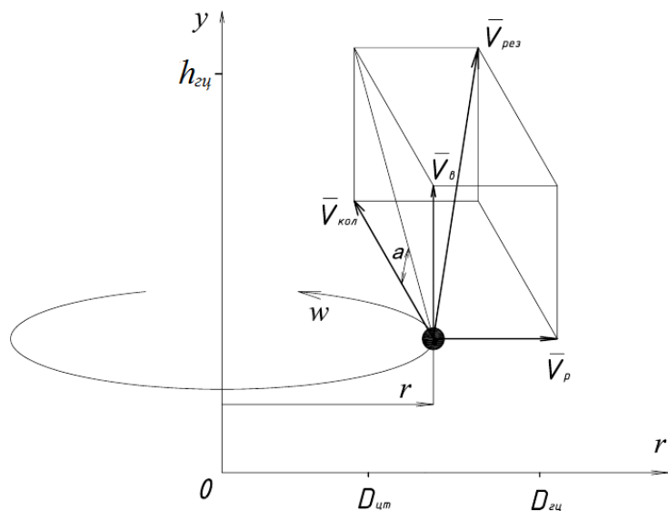
Рис. 2. Векторна діаграма швидкостей руху повітряного потоку в циклонному пристрої: y – напрямком вертикалі циклонного пристрою; h_{\text{ц}} – висота циліндру; \bar{V}_{\text{г}} – швидкість частинки в напрямку вертикалі; \bar{V}_{\text{кол}} – швидкість руху частинки по колу; \bar{V}_{\text{р}} – швидкість руху частинки в радіальному напрямку; \bar{V}_{\text{рез}} – результуючий вектор швидкості руху частинки в каналі циклону; \alpha – кут підйому гвинтової лінії перегородки; r – координата радіусу обертання частинки; D_{\text{ц}} – діаметр циліндру; D_{\text{цт}} – діаметр центральної труби; \omega – кутова швидкість обертання повітряного потоку
