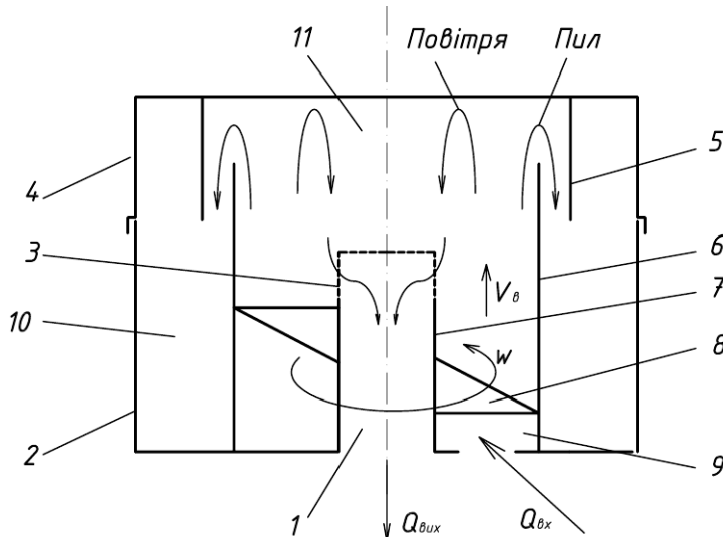
Рис. 1. Схема руху повітряного потоку в циклонному пристрої пилососа:
