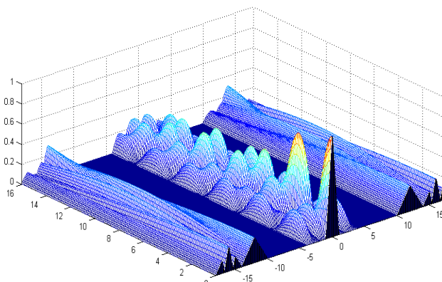
Рис. 3. ФН послідовності двох пакетів комплементарних кодів
