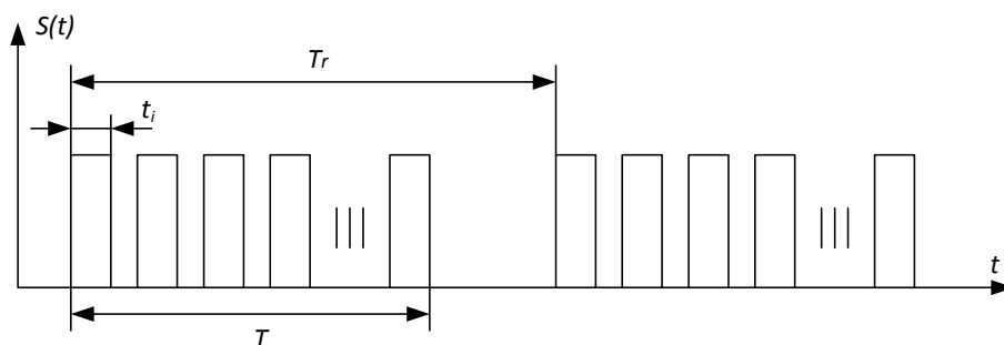
Рис. 1. Послідовність когерентних імпульсів
