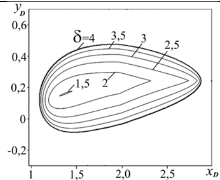
Рис. 6. Ізолінії коефіцієнтів нерівномірності руху \delta
