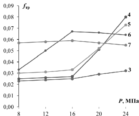
Рис. 2 – Залежність коефіцієнту тертя від контактної навантаження в парі тертя «бронза БрАЖ 9-4 - сталь 45» з мастильною композицією «олива І-20А + тіоамід» ( t = 25\text{ }^{\circ}\text{C} , \tau = 3,00\text{ год} )
