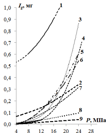
Рис. 1 – Залежність зношення від контактної навантаження в парі тертя «бронза БрАЖ 9-4 - сталь 45» з мастильною композицією «олива І-20А + тіоамід» ( t = 25\text{ }^{\circ}\text{C} , \tau = 3,00\text{ год} )
