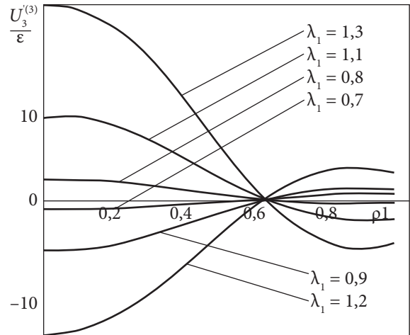
Рис. 2. Переміщення U'_3/\varepsilon при z_i = 0
