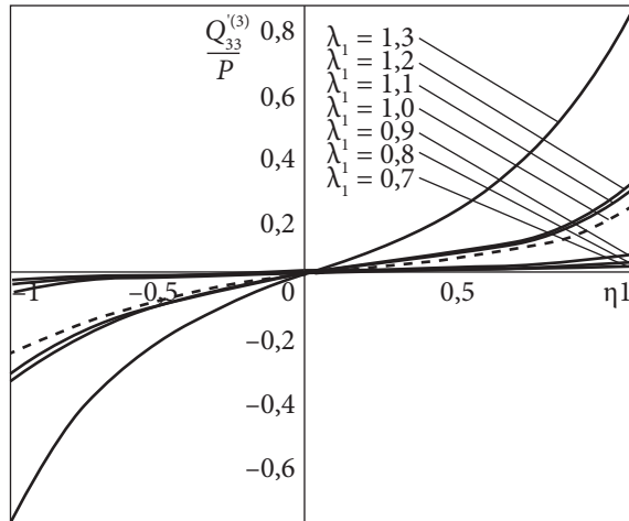
Рис. 1. Нормальні напруження Q'_{33}/P вздовж циліндричного штамп
