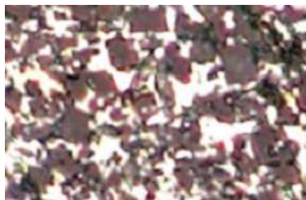
Рис. 2. Микроструктура алюмокомпозита с муллитовым наполнителем.
