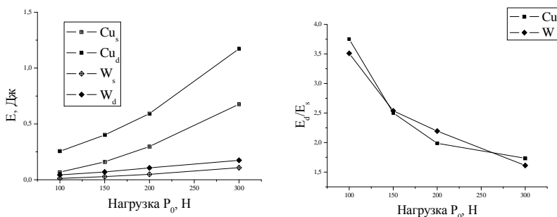
Рис. 2. Изменение зависимости энергии деформации (а) и отношения E_d/E_s (б) для Cu, W при увеличении постоянной нагрузки P_0 .
