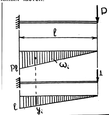
Рис.1. Расчётная схема определения прогиба навигационного устройства и интрамедуллярного фиксатора: а) консольный стержень с приложенной боковой изгибающей силой; б) эпюра изгибающего момента от внешней нагрузки; в) единичная безразмерная сила, приложенная в сечении, где определяется прогиб; г) эпюра изгибающего момента от единичной силы
