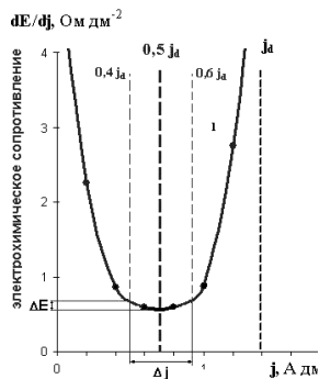
Рис.2 Зависимость электрохимического сопротивления от плотности тока
