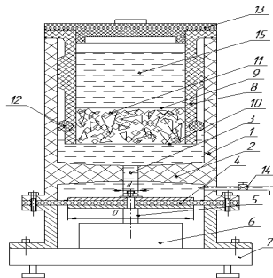
Рис. 2 – Конструктивна схема вібраційного пристрою
