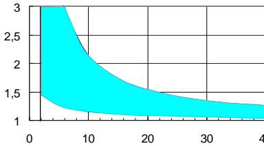
Рис.2. Обобщенная зависимость \sigma_{\delta,max}^* / \sigma_{\delta,изм,max} от объема выборки z_\delta
