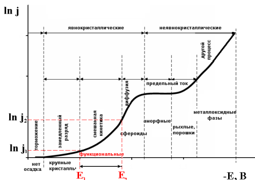
Рис.1. Взаимосвязь электрохимической кинетики и электроосаждения металлов
