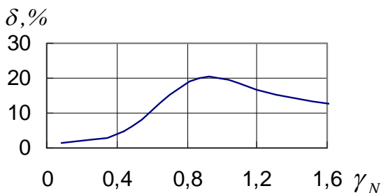
Рис.3. Зависимость логарифмического декремента колебаний модели от силы прижатия вставок при импульсном возбуждении
