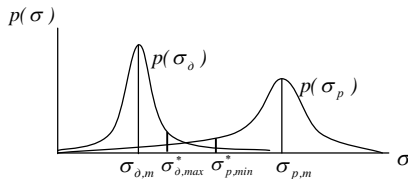
Рис.1. Плотности распределений p(\sigma_d) и p(\sigma_p)
