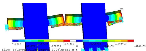
Рис.1. а) Элементарная 3D модель лопаток с отодвинутыми от трактовых полок демпферными вставками; б) деформации модели
