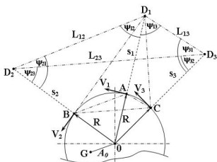
Рис. 2. Определение радиуса R ротора
