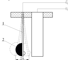
1 – консольна балочка; 2 - вантаж Рисунок 2 – Датчик вібрацій
