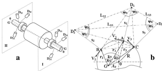
Рис. 1. Определение положения оси вращения и оси симметрии ротора
