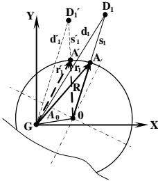
Рис. 3. Смещение датчика при измерении вибрации ротора
