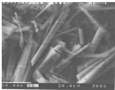
Рис. 1. Типичная структура кристаллов на основе муллита
