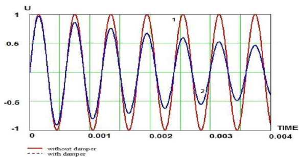
Рис.2. Начальные периоды изменения перемещений контрольного узла модели по времени: 1) без вставок, 2) со вставками
