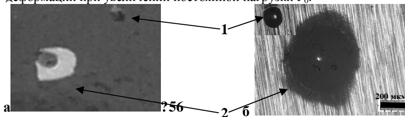
Рис.1. Вид отпечатка индентора на образце (а) покрытия и (б) монокристалла W при статическом (1) и динамическом (2) режиме нагружения. P_0=100Н ;
