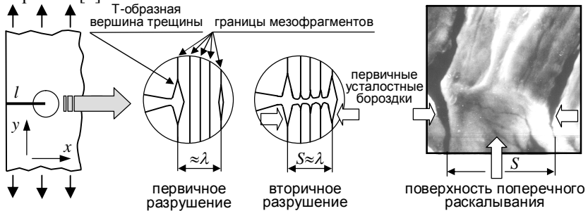
Рис.1. Схема действия микромеханизма периодического расслаивания-разрыва (поперечное сечение фронта трещины) и электронная фрактограмма бороздчатой структуры, расколовшейся в поперечном направлении к бороздкам
