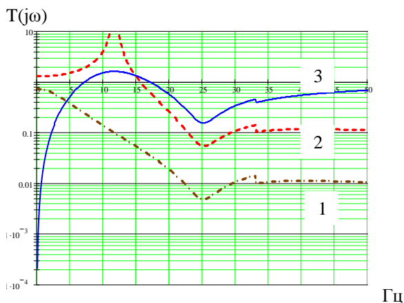
Рис 1. Передаточная функция при моделировании системы виброизоляции с настройкой на частоту 25 Гц на различные типы основания
